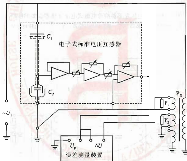
图5 用电子式标准电压互感器检验电压互感器误差线路
