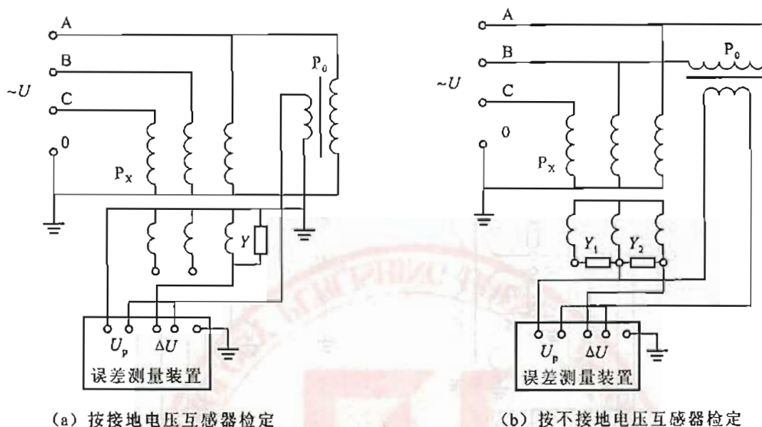
图4 三相五柱电压互感器误差检验线路
