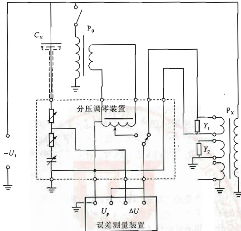
图6 用电容分压器检验电磁式电压互感器的线路
