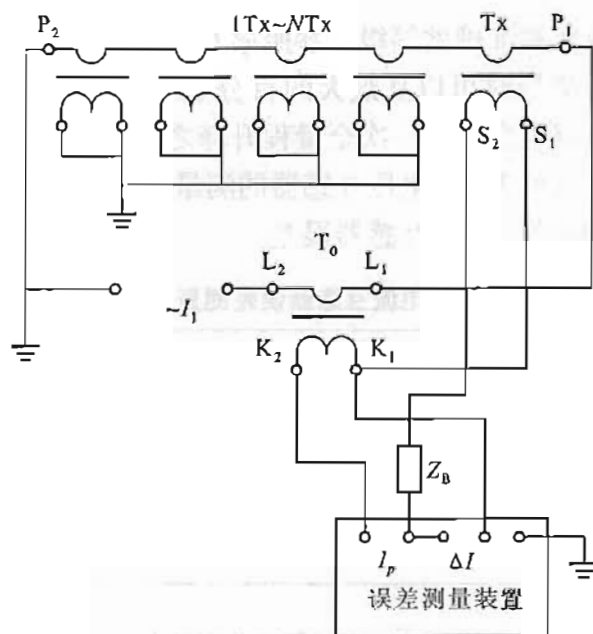
图 1 电流互感器误差测量接线
