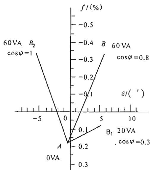
图 D1 电压互感器二次负荷误差计算图
